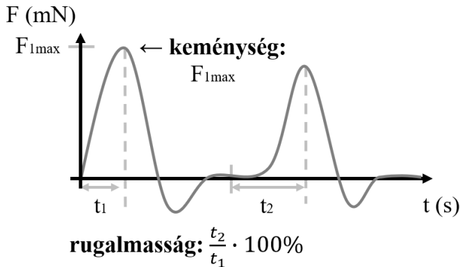
9. ábra: Az erő-idő görbéről meghatározott mechanikai paraméterek
